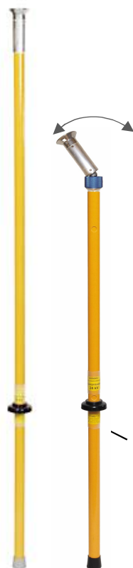
Manöverstång MRS 24 max 24 kV, l=1,6m
